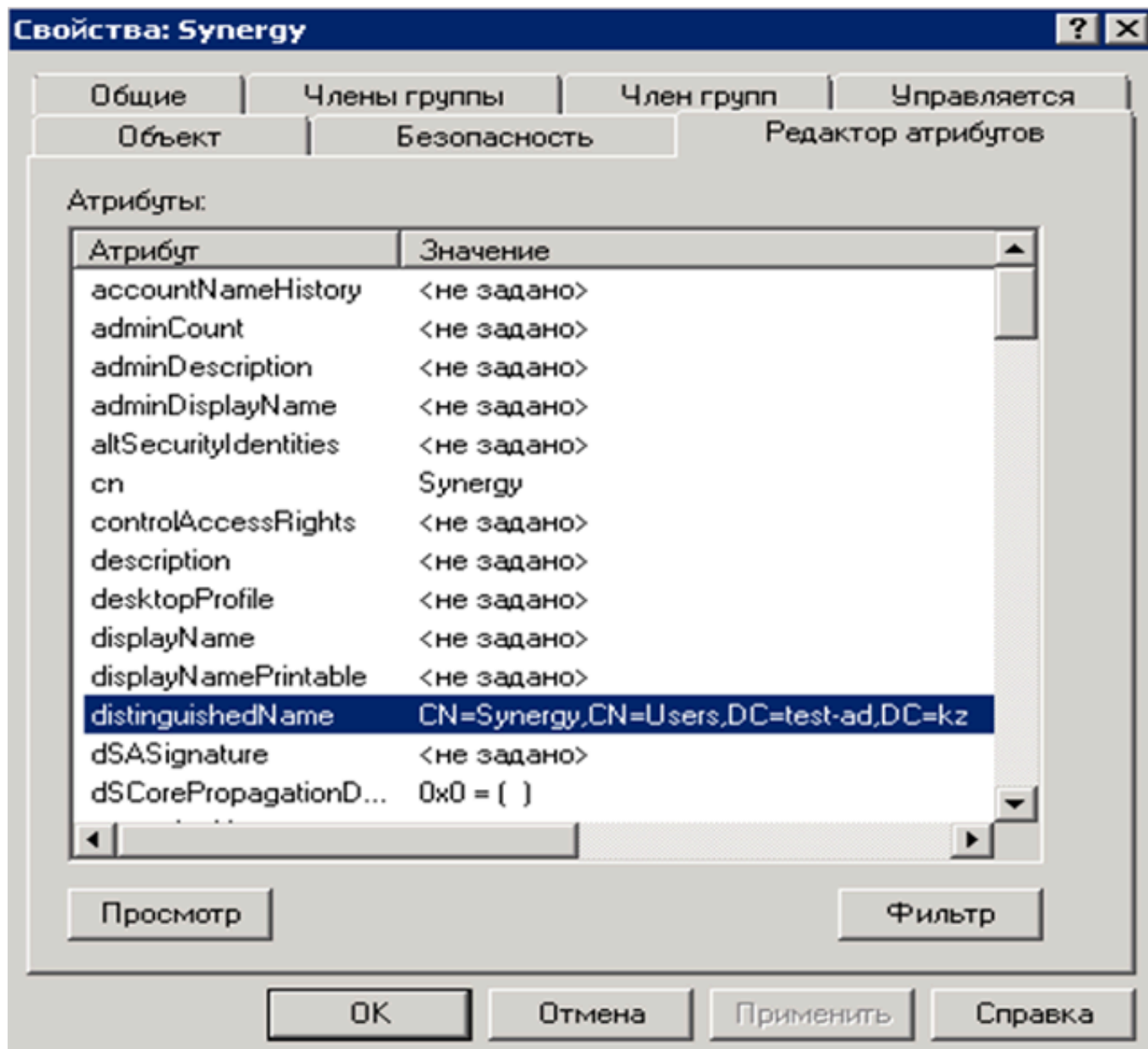
Figure 7.30: Рисунок 3
