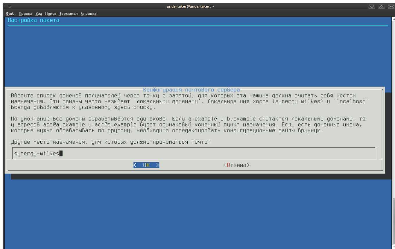
Figure 7.36: Другие назначения
