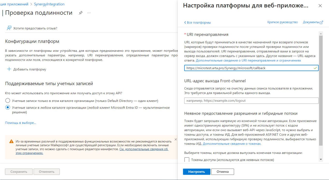
Figure 7.76: URL редиректа
