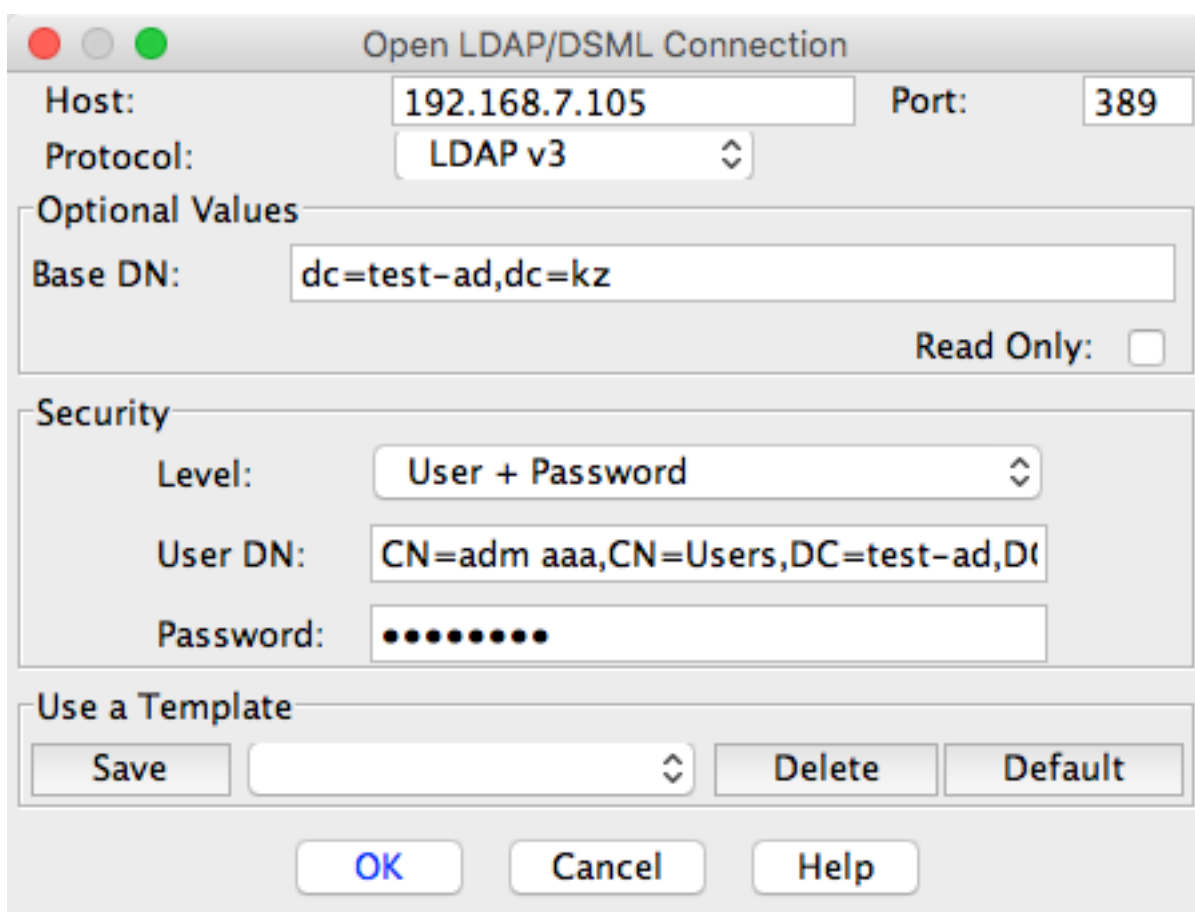
Figure 7.21: Рисунок 1
