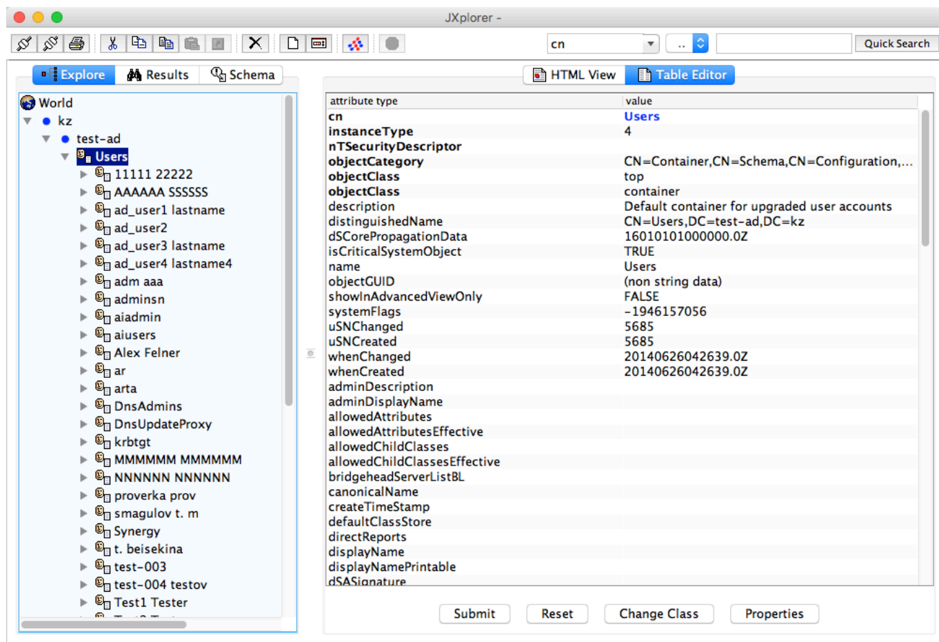
Figure 7.18: Рисунок 2
