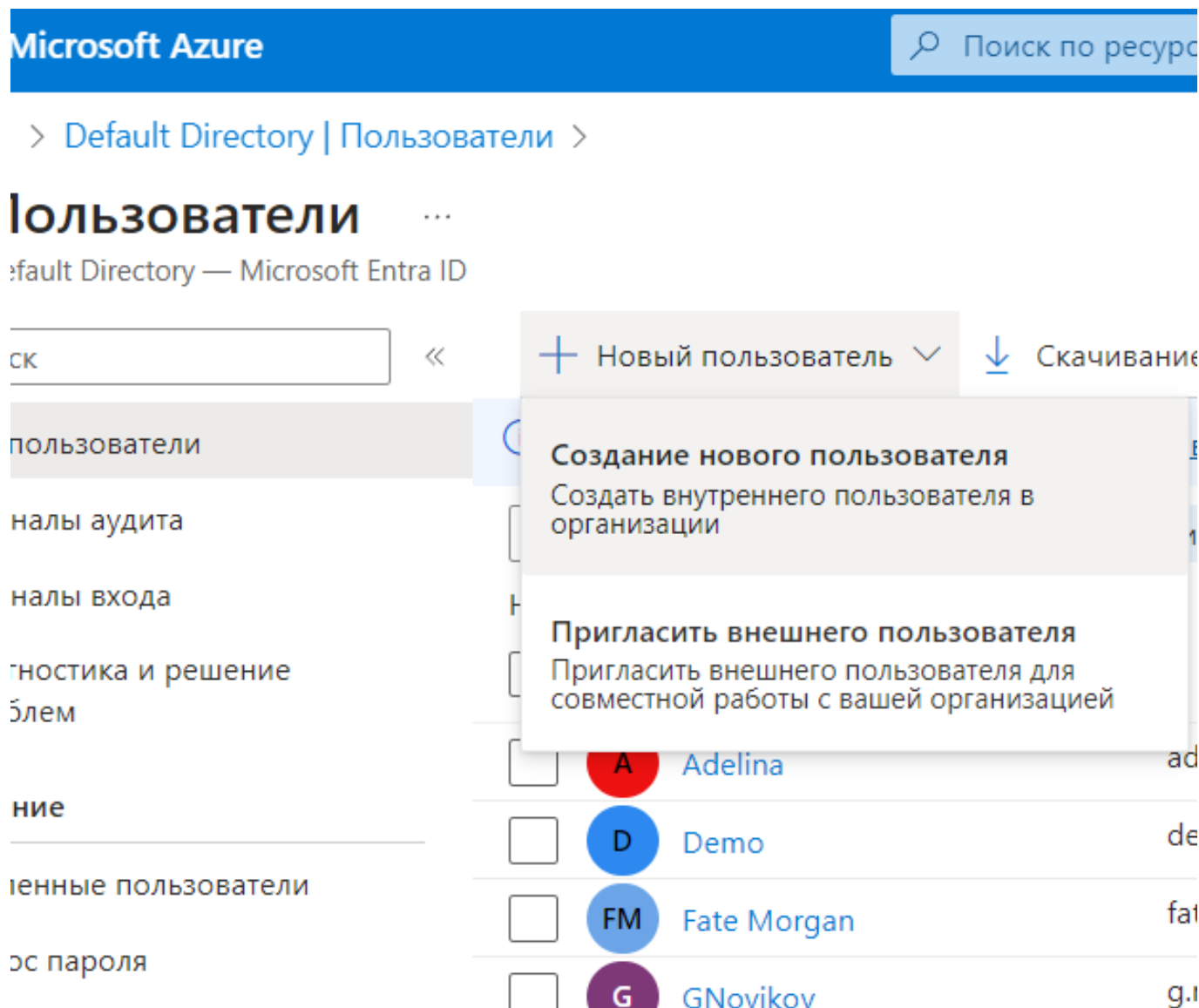
Figure 7.83: Новый пользователь
