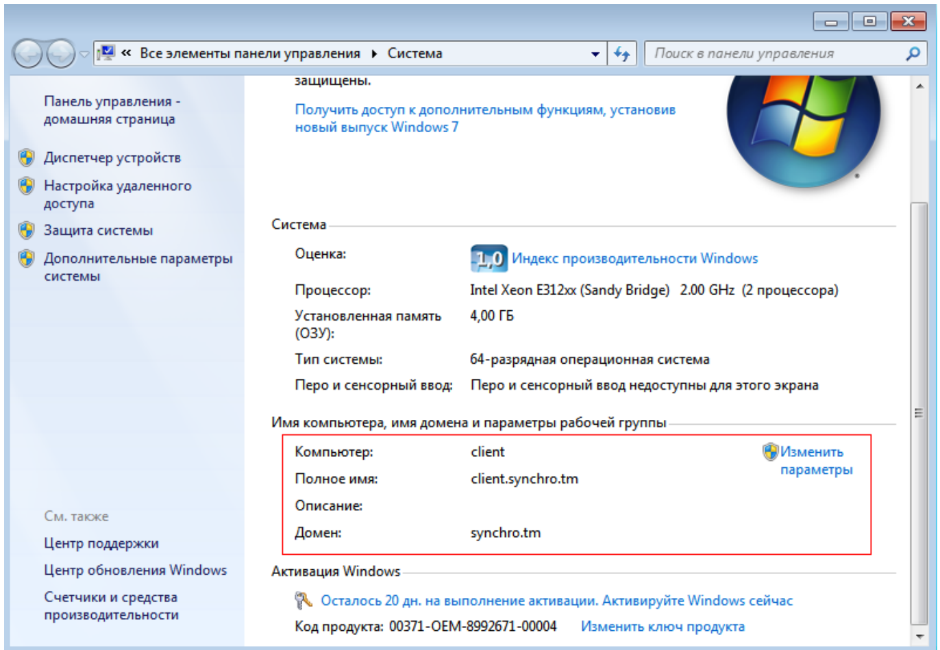
Figure 7.52: Свойства компьютера-клиента
