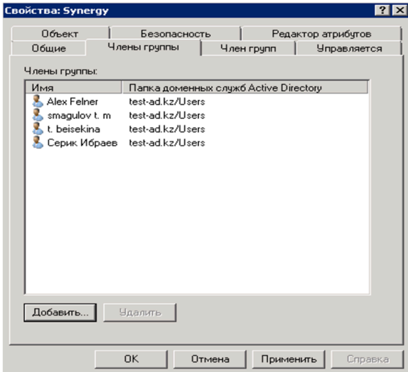
Figure 7.29: Рисунок 2
