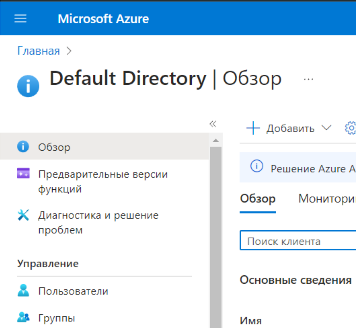
Figure 7.82: Пользователи
