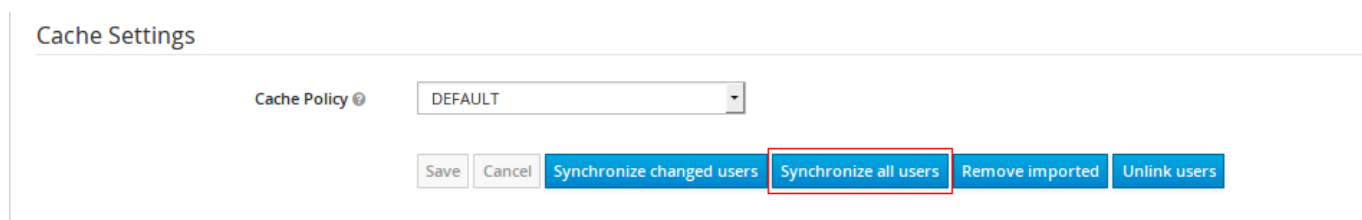
Figure 7.67: Синхронизация пользователей
