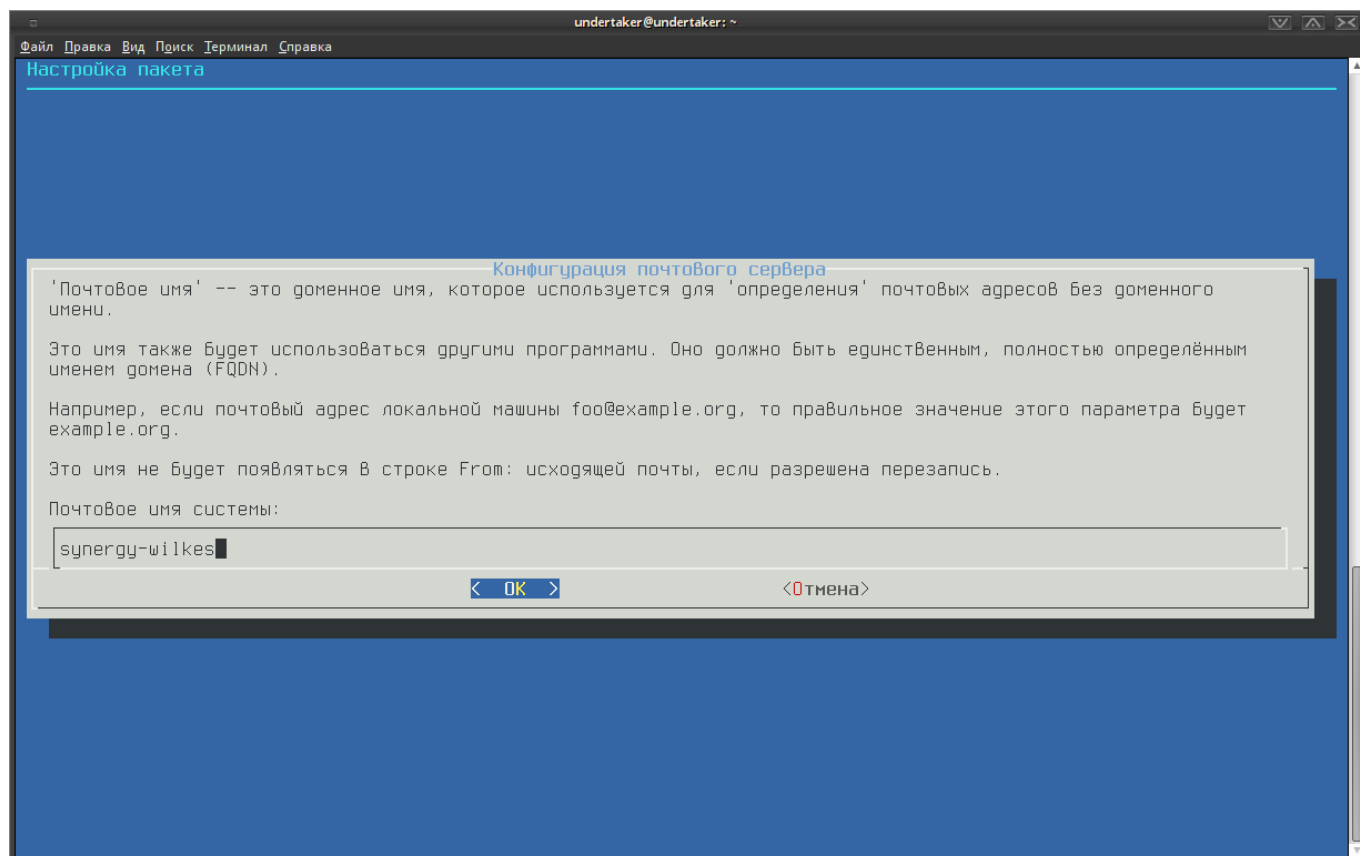
Figure 7.34: Почтовое имя
