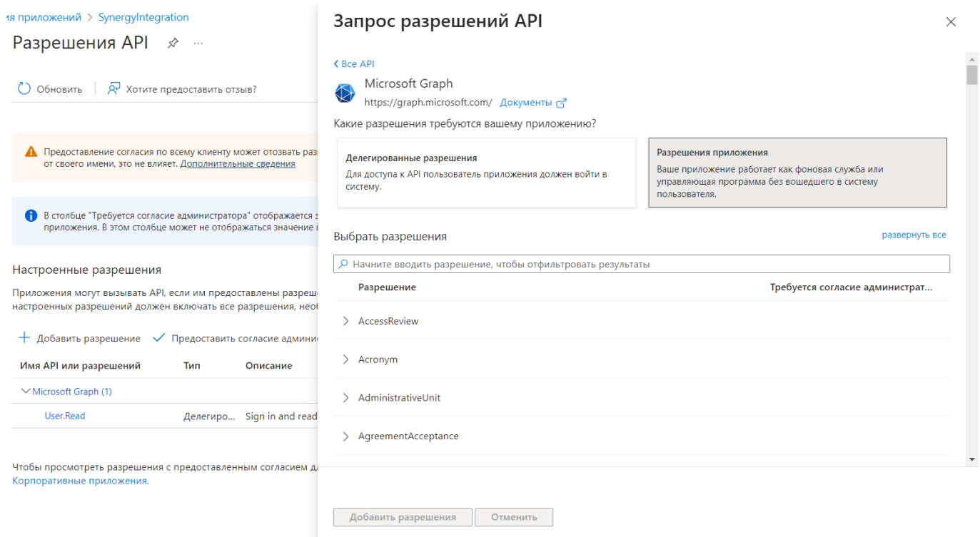
Figure 7.77: Разрешения API
