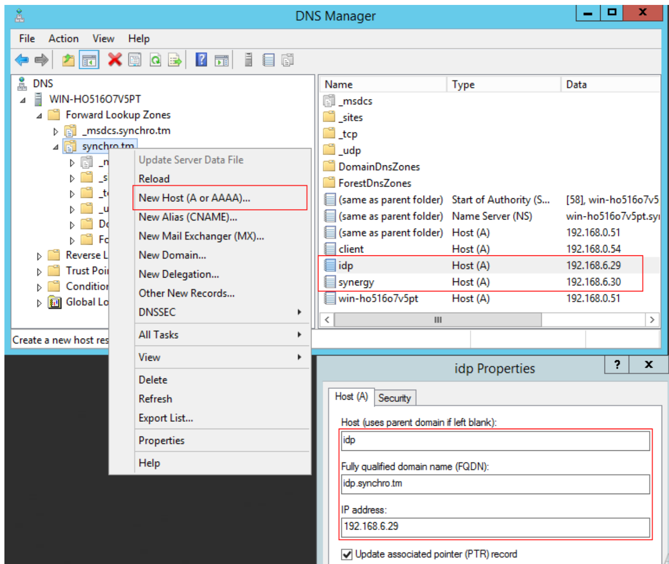
Figure 7.50: Добавление хостов
