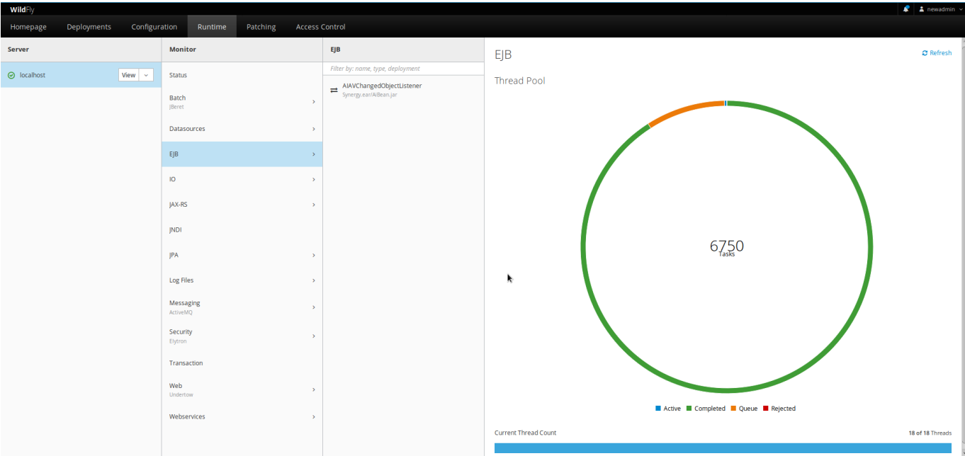
Figure 7.14: Потоки EJB
