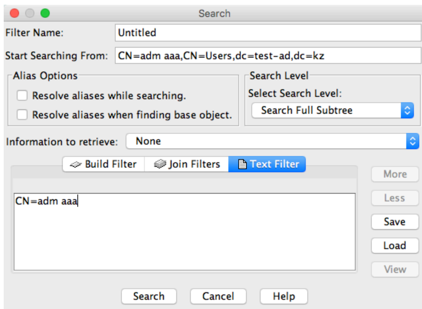
Figure 7.19: Рисунок 3
