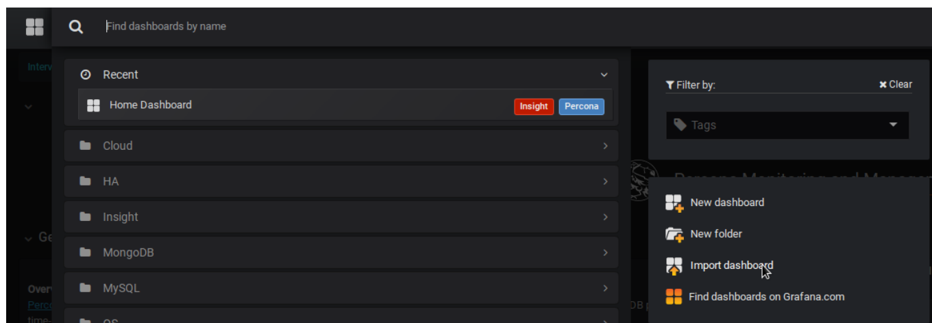
Figure 6.3: Импорт дашборда
