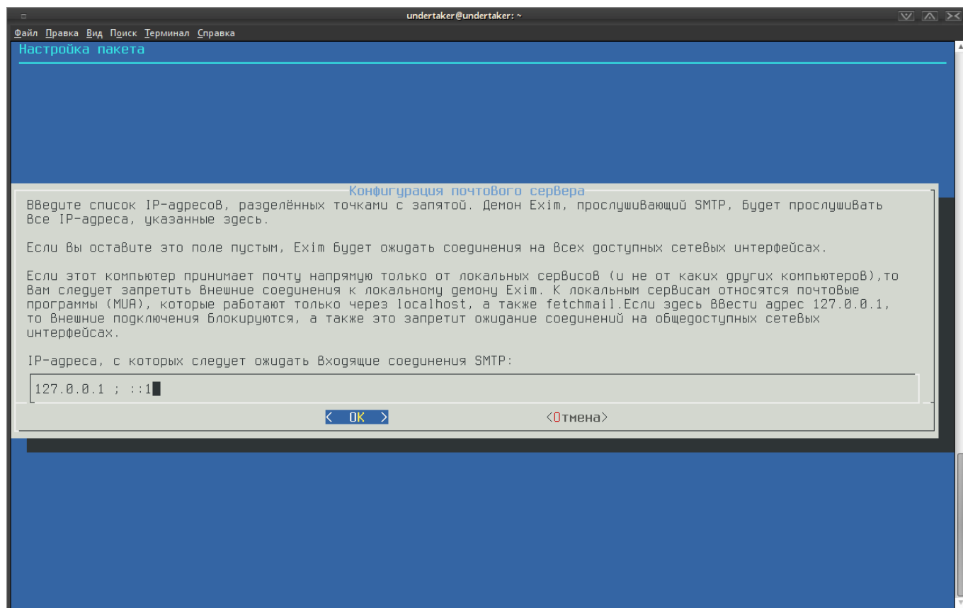
Figure 7.35: Входящие соединения
