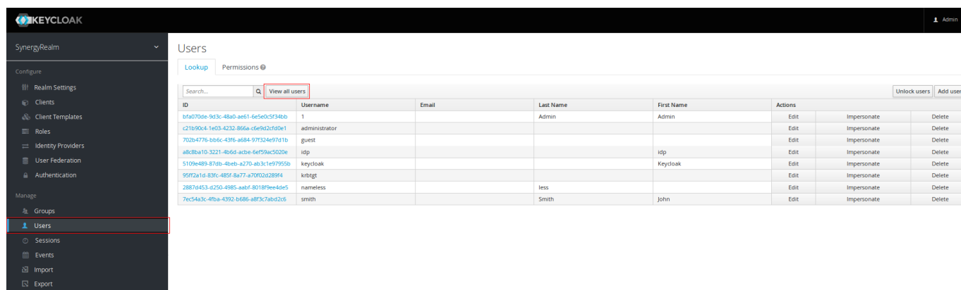
Figure 7.68: Просмотр пользователей
