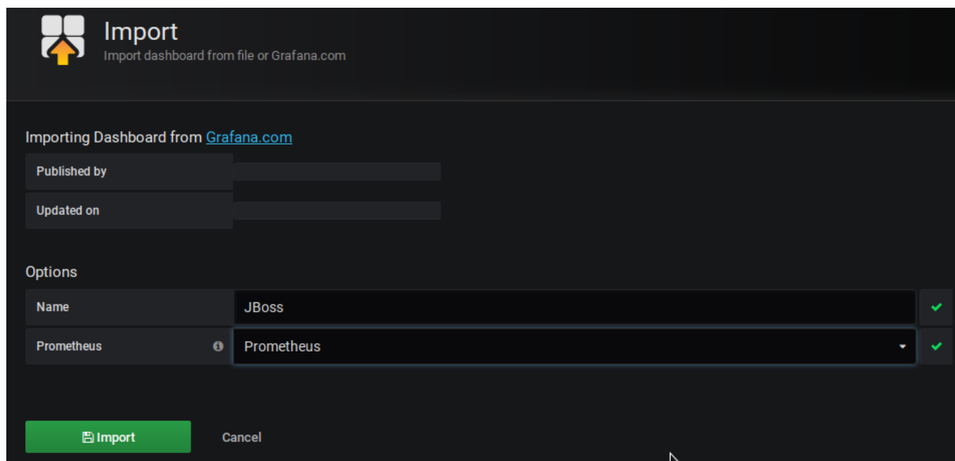
Figure 6.4: Выбор json-файла
