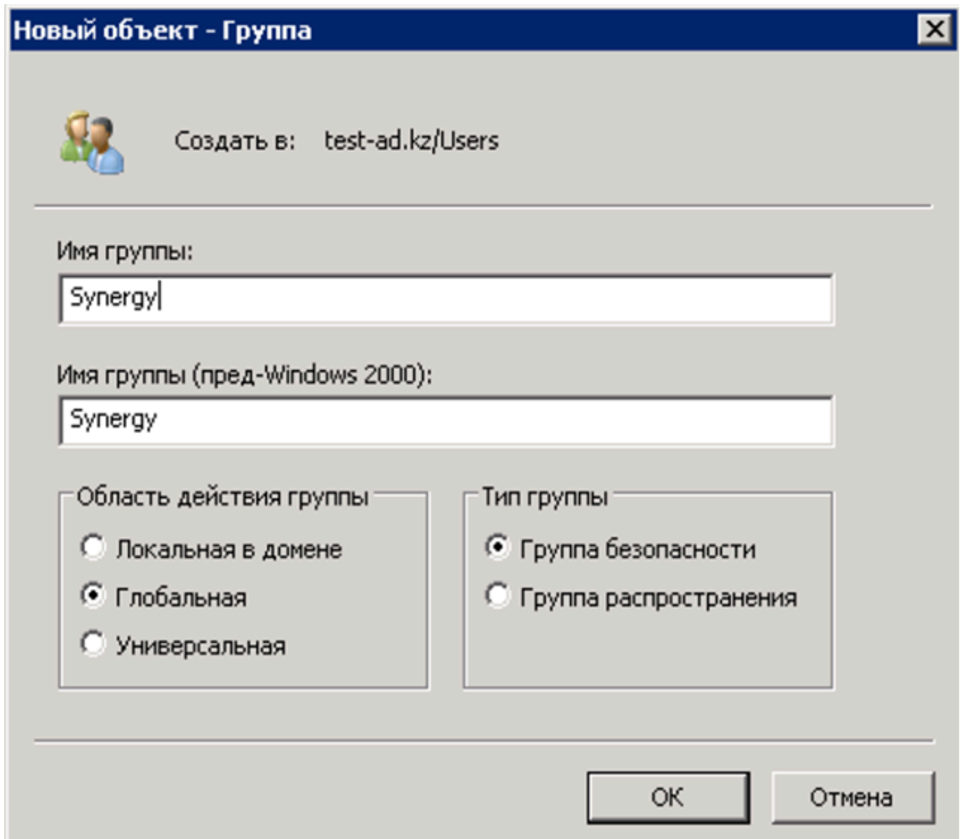
Figure 7.31: Рисунок 4
