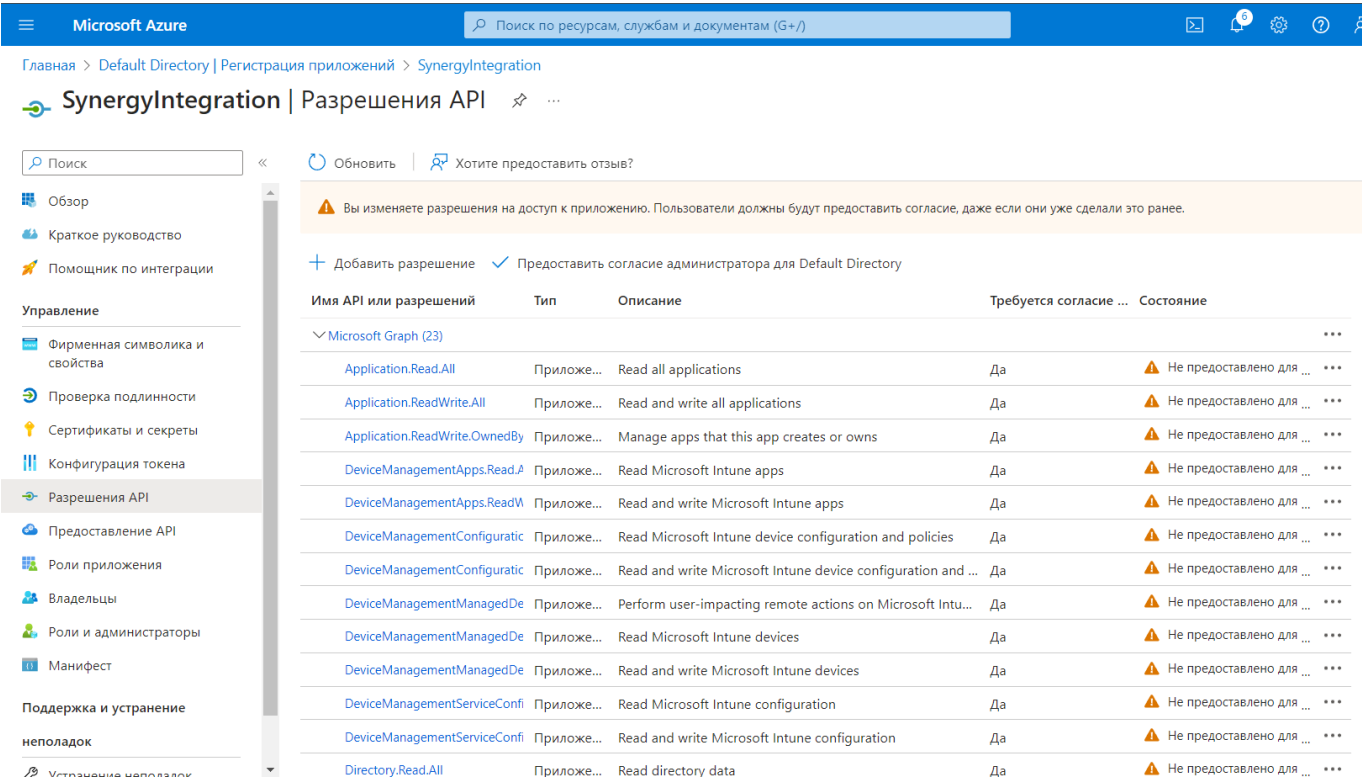
Figure 7.79: Согласие администратора
