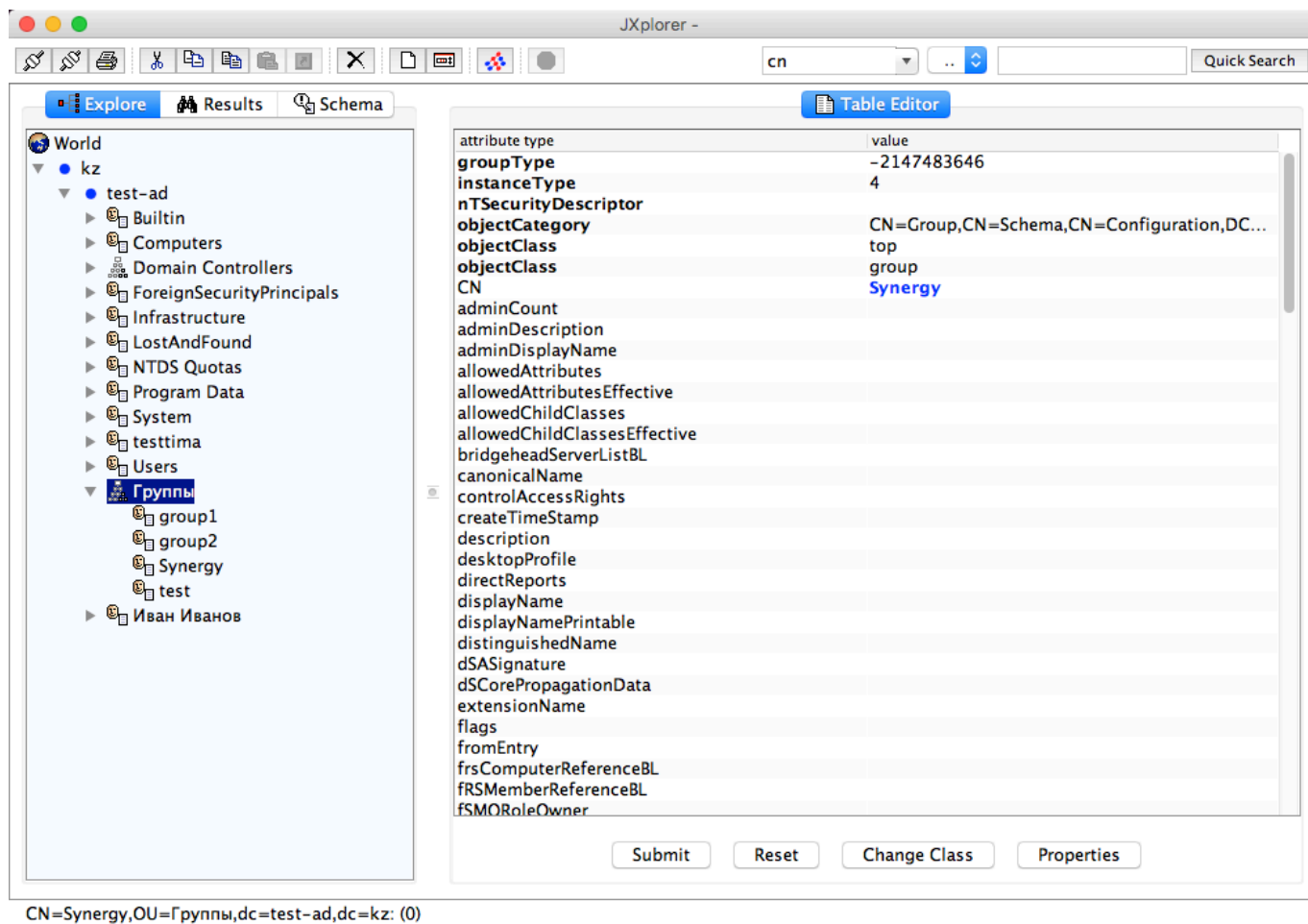
Figure 7.25: Рисунок 5
