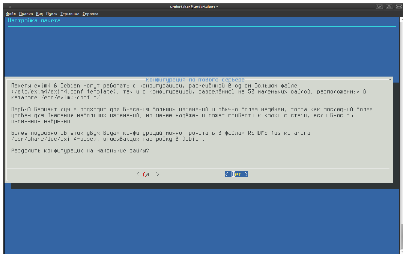
Figure 7.43: Разделение конфигурации
