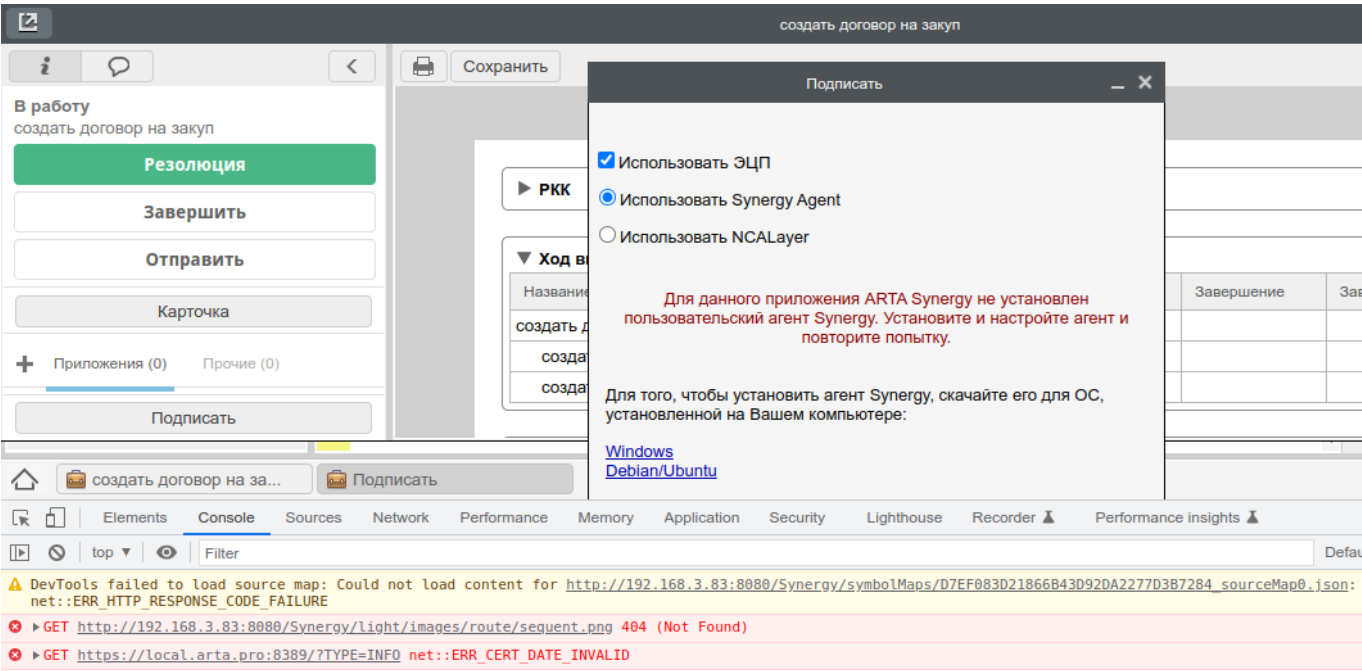
Figure 5.2: Невалидный сертификат
