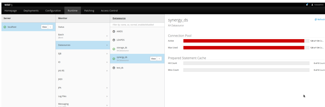
Figure 7.13: Нехватка соединений
