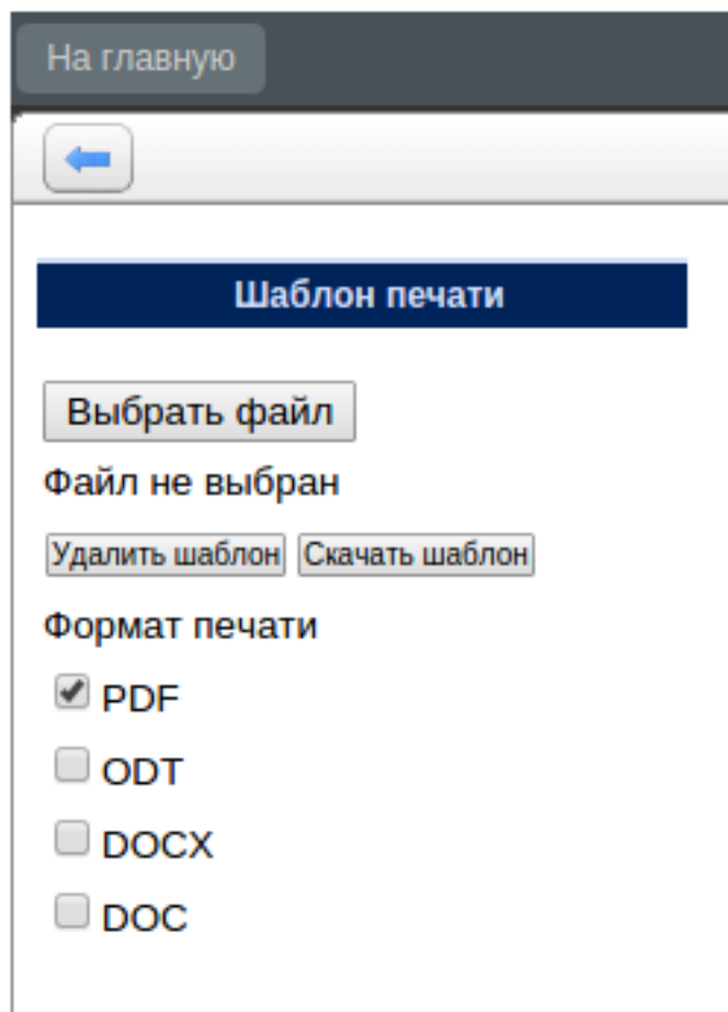
Рис. 13.5: Добавление шаблона
