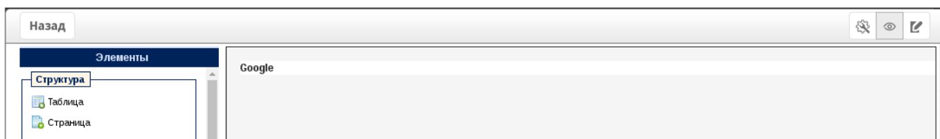
Рис. 3.70: Активная ссылка
