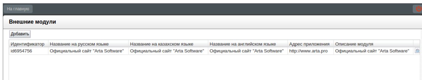
Рис. 11.11: Внешние модули
