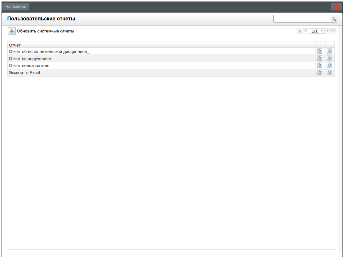
Рис. 12.6: Окно отчётов
