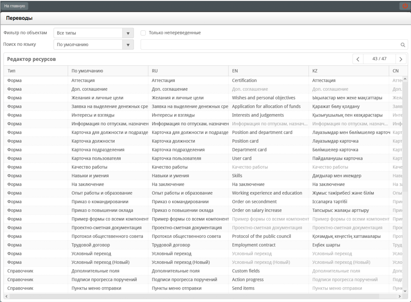
Рис. 11.3: Переводы
