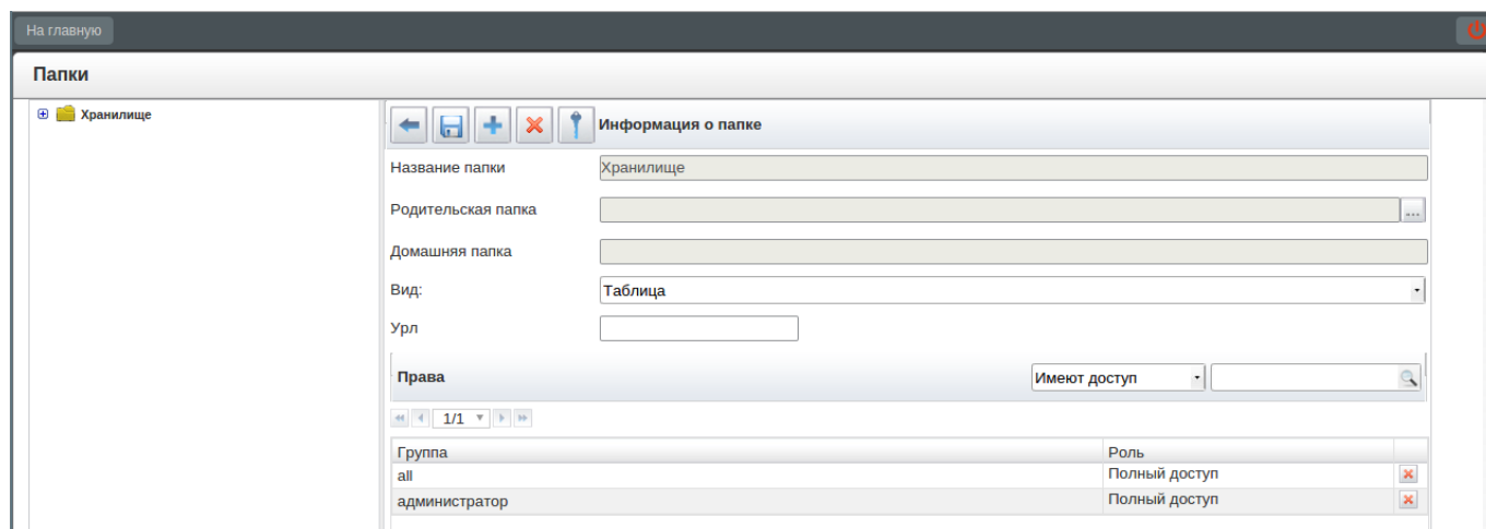
Рис. 7.1: Раздел «Папки»
