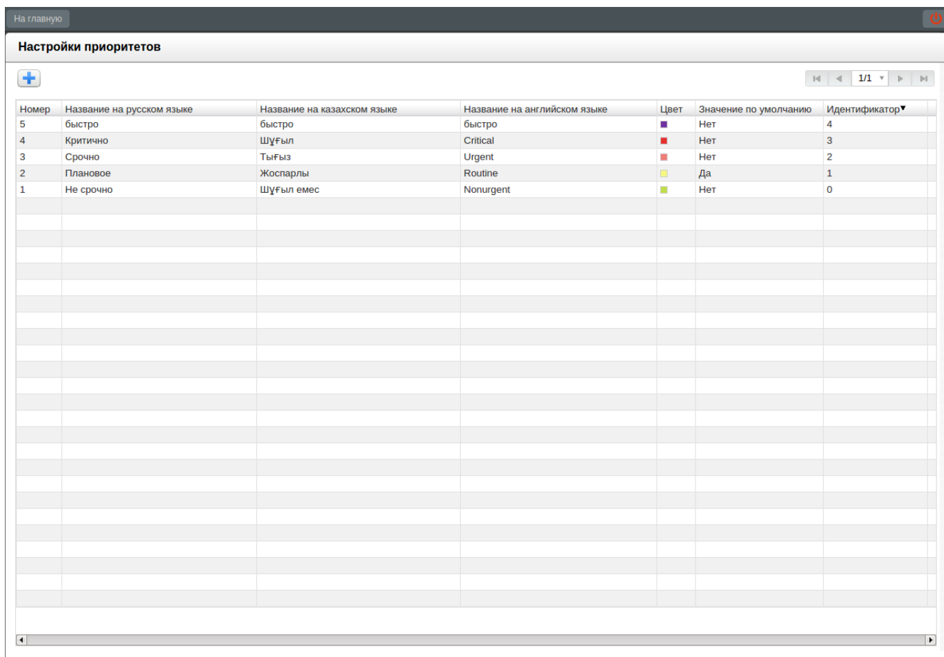
Рис. 4.23: Настройки приоритетов
