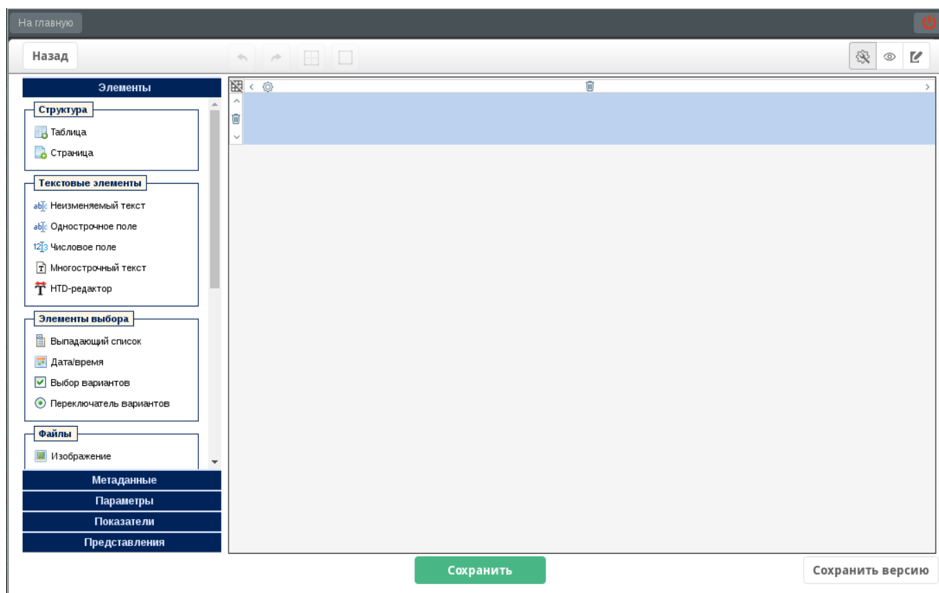
Рис. 3.5: Редактор форм
