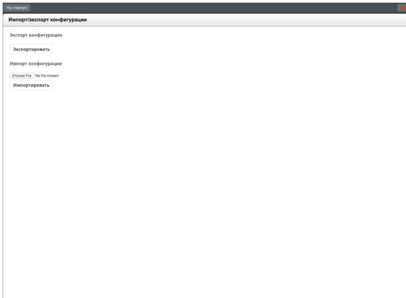
Рис. 11.18: Импорт/Экспорт конфигурации
