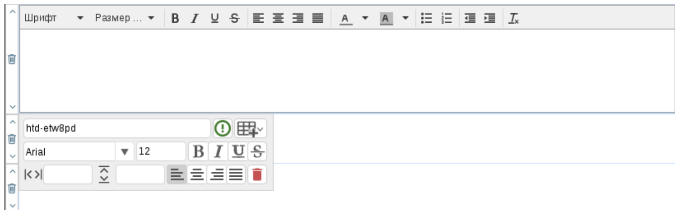
Рис. 3.20: Компонент «HTD-редактор»
