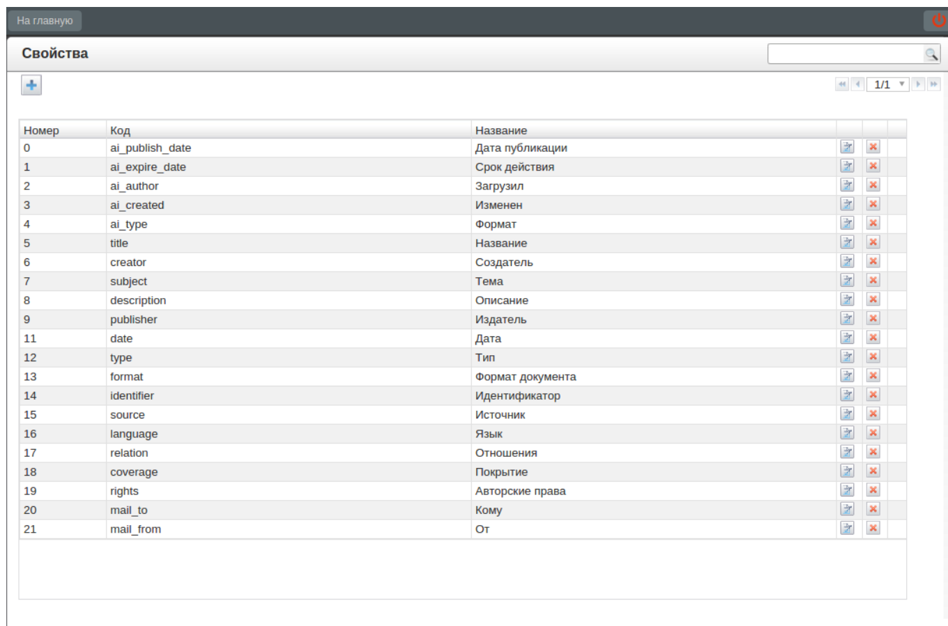
Рис. 7.11: Свойства
