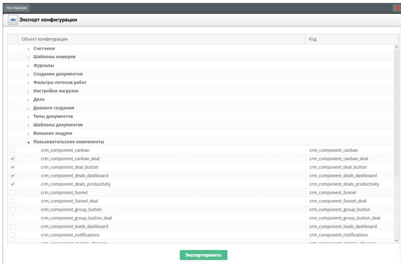
Рис. 11.19: Экспорт конфигурации
