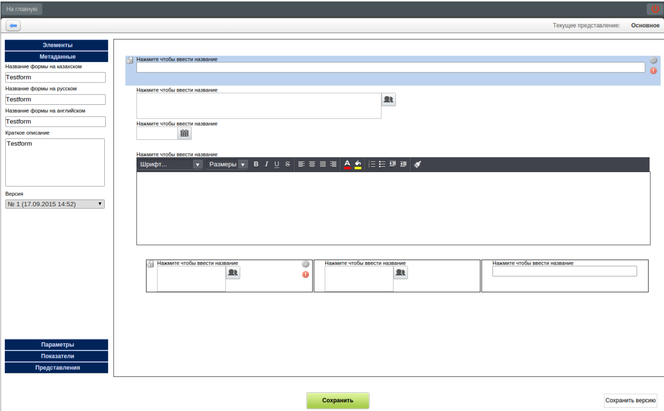
Рис. 13.1: Создание формы
