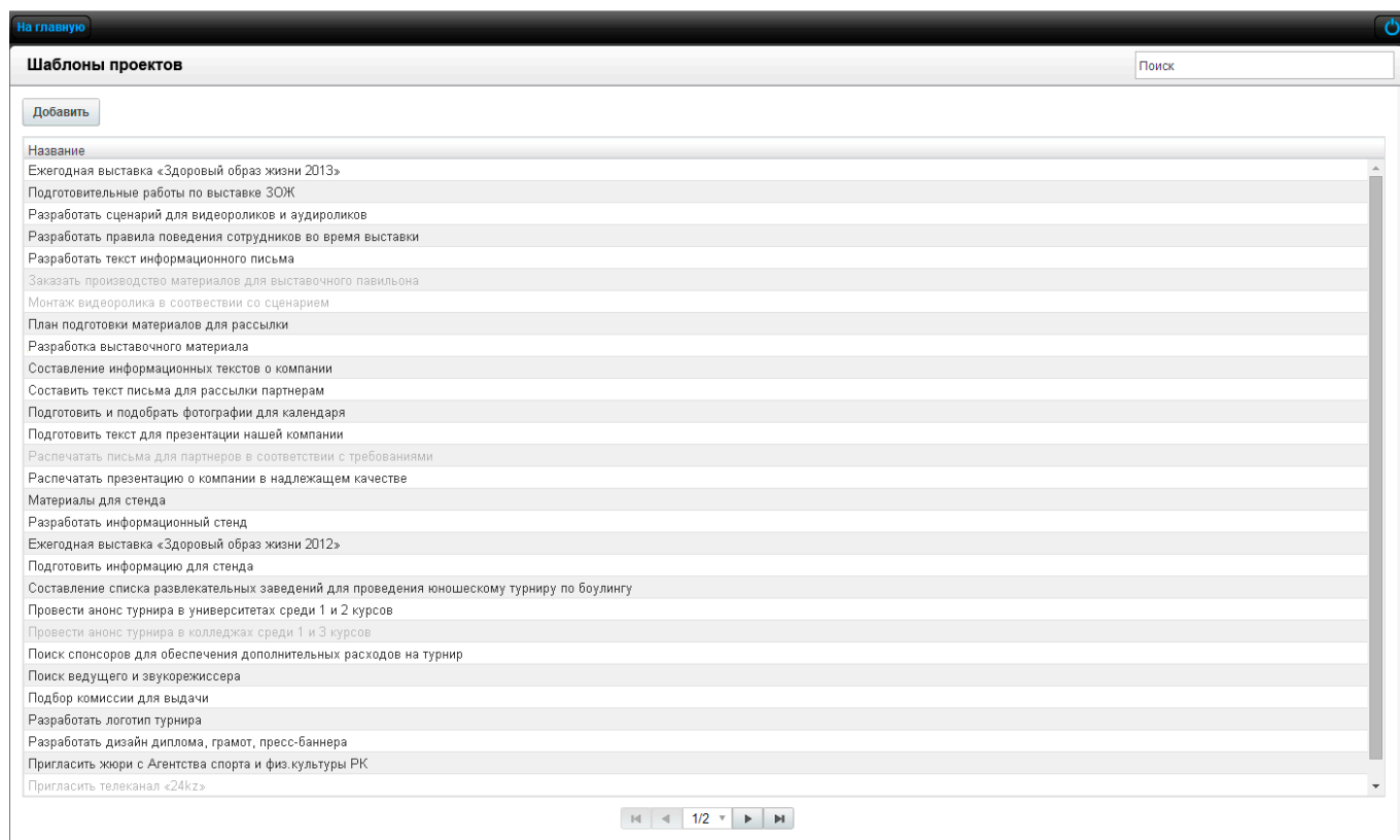
Рис. 6.4: Шаблоны проектов
