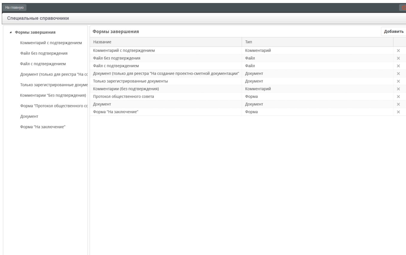
Рис. 3.142: Специальные справочники
