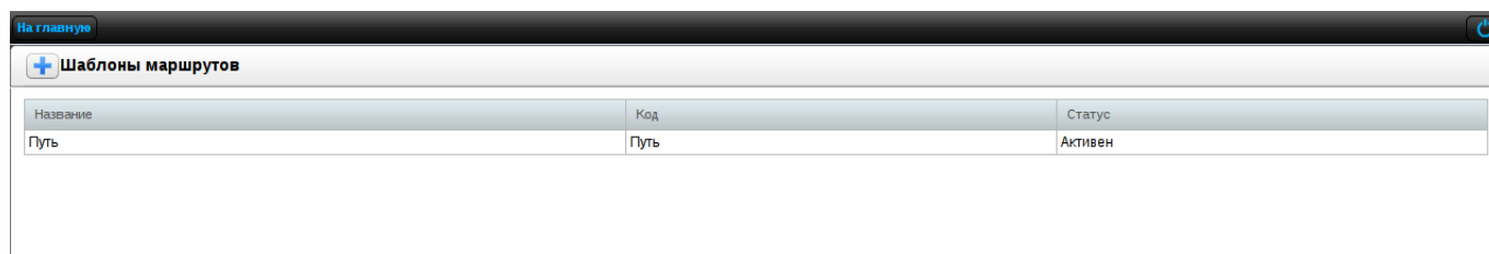
Рис. 3.116: Шаблоны маршрутов
