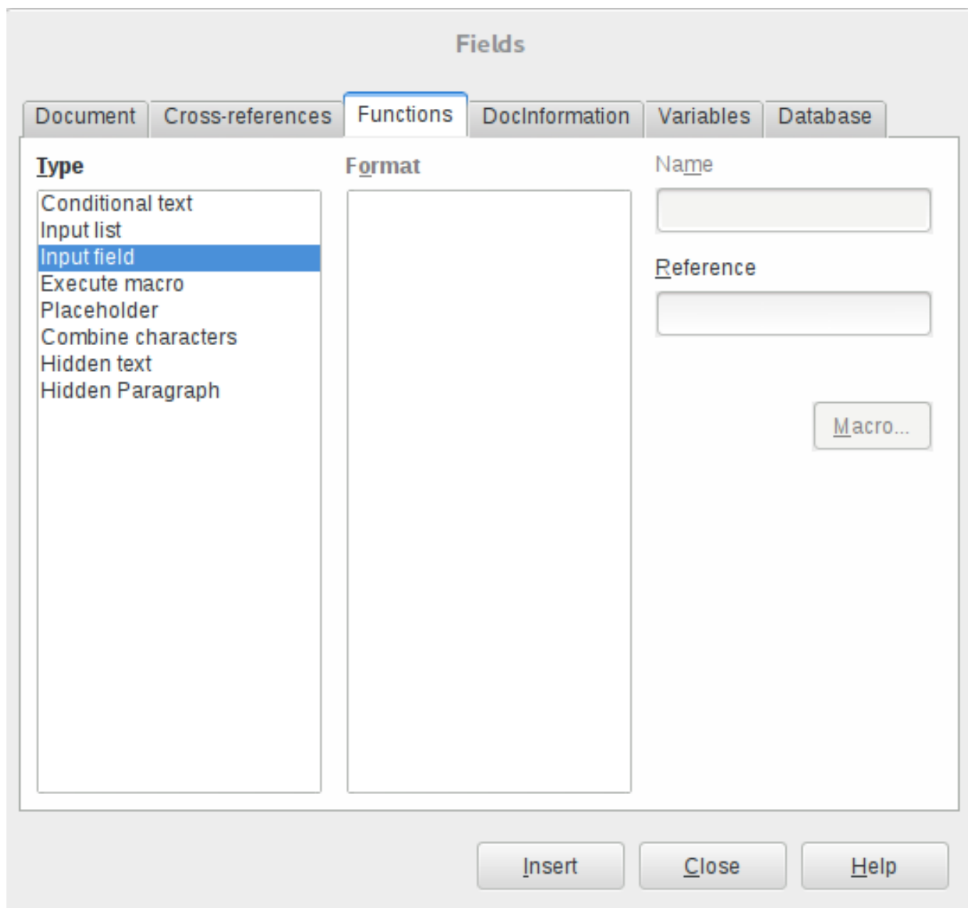
Рис. 13.2: Вставка компонента-1
