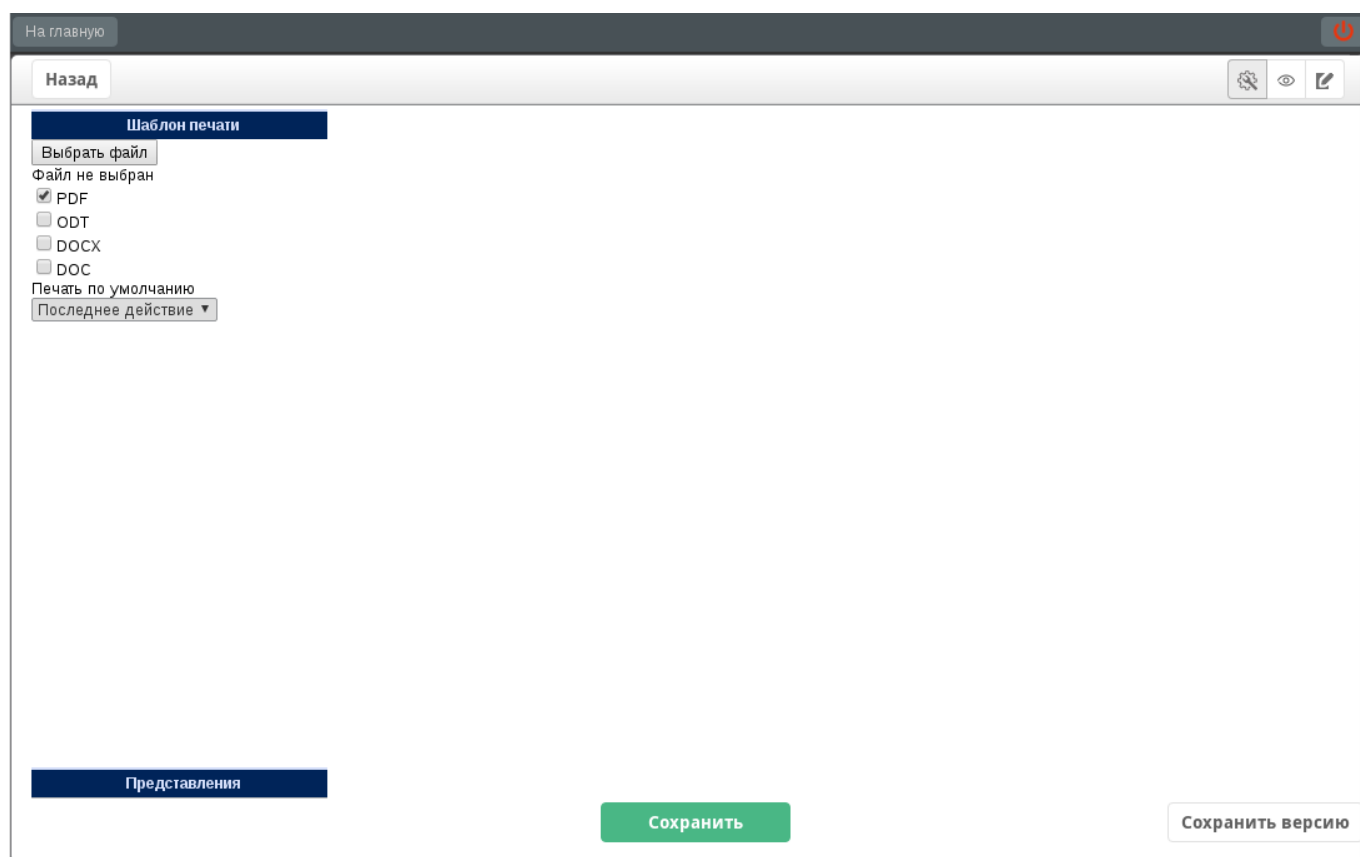
Рис. 3.80: Печатное представление
