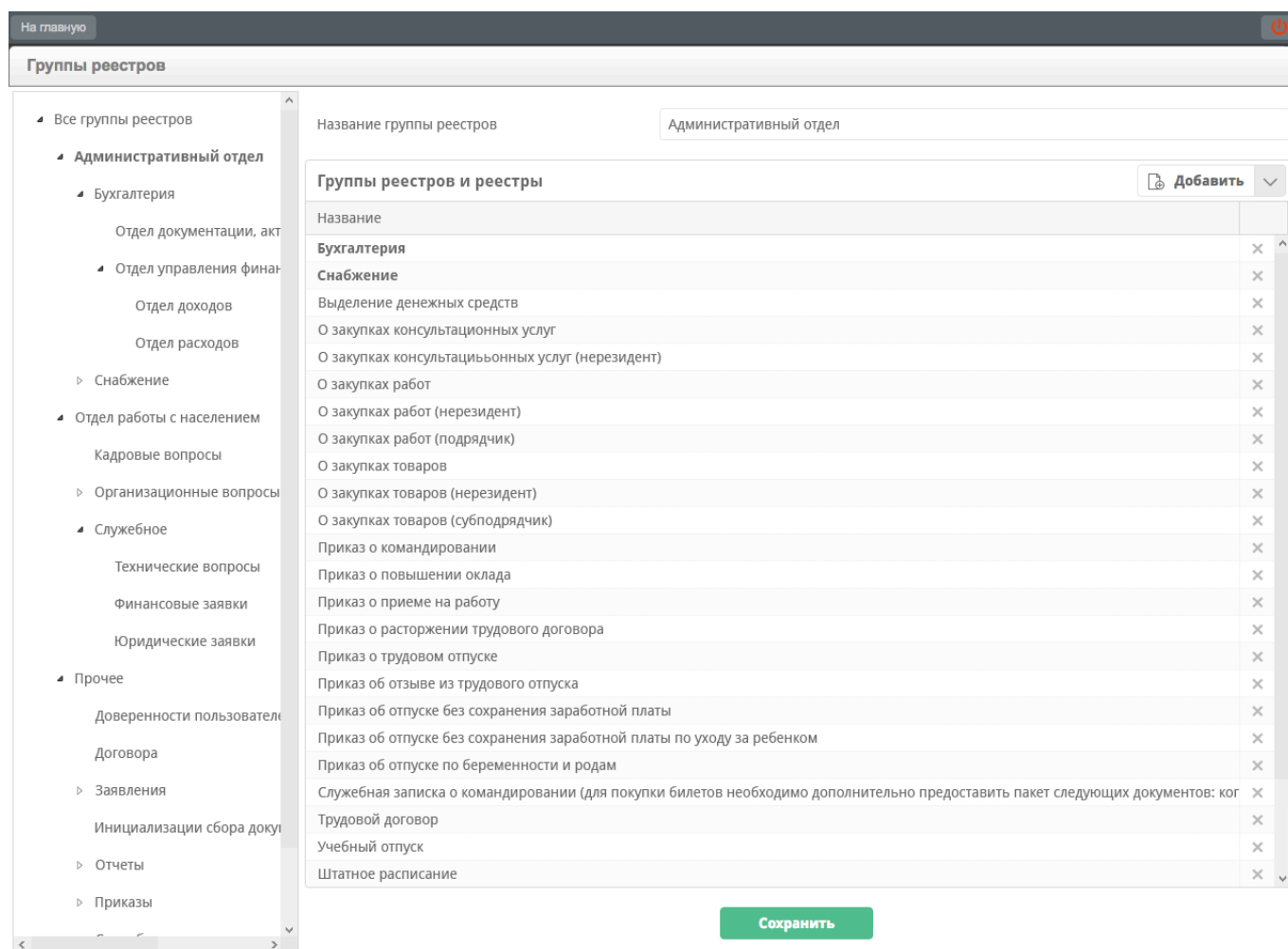
Рис. 3.114: Группы реестров
