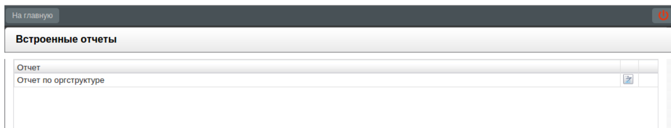
Рис. 12.1: Встроенные отчеты
