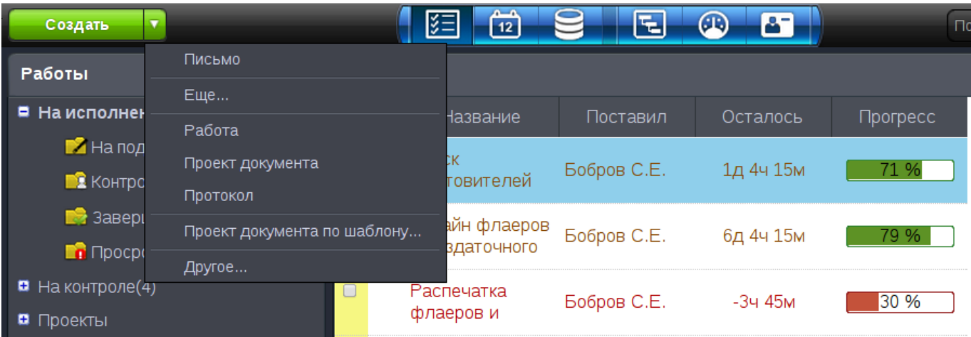
Рис. 10.11: Кросс-модульная кнопка
