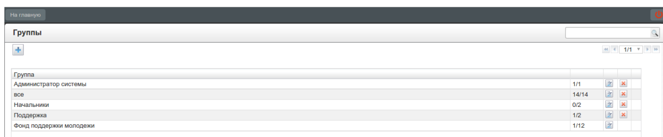
Рис. 7.4: Раздел «Группы»
