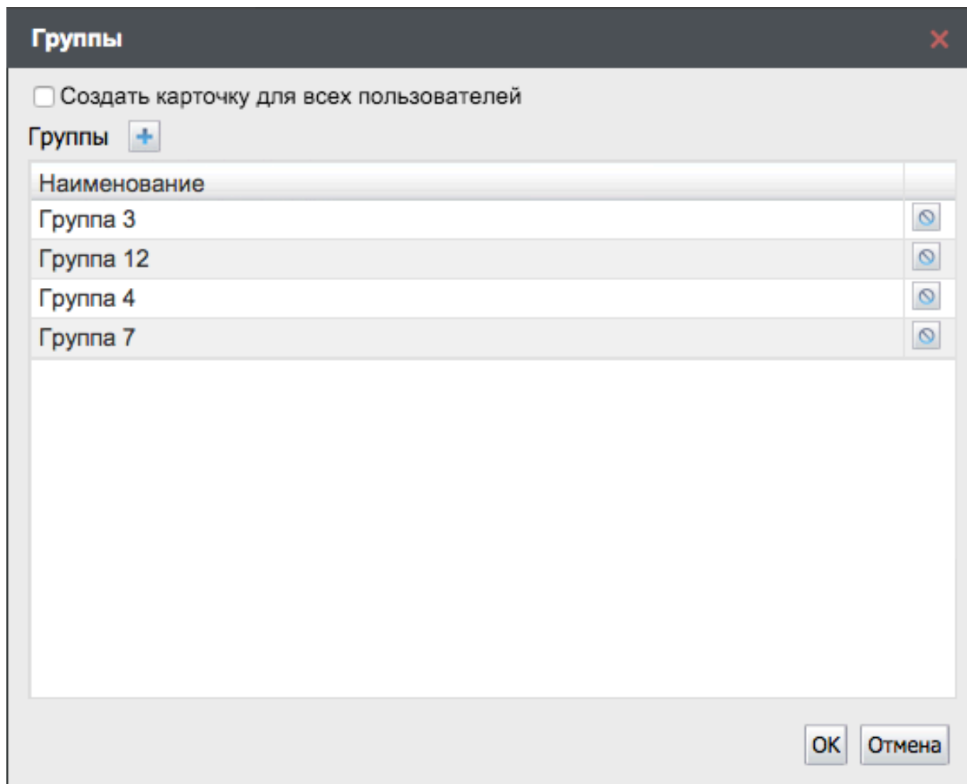
Рис. 5.9: Группы
