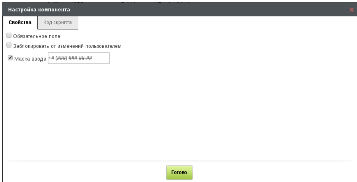
Рис. 3.54: Маска ввода
