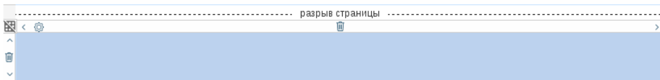
Рис. 3.16: Компонент Страница
