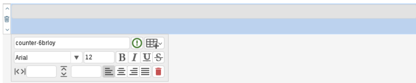
Рис. 3.36: Компонент «Номер»
