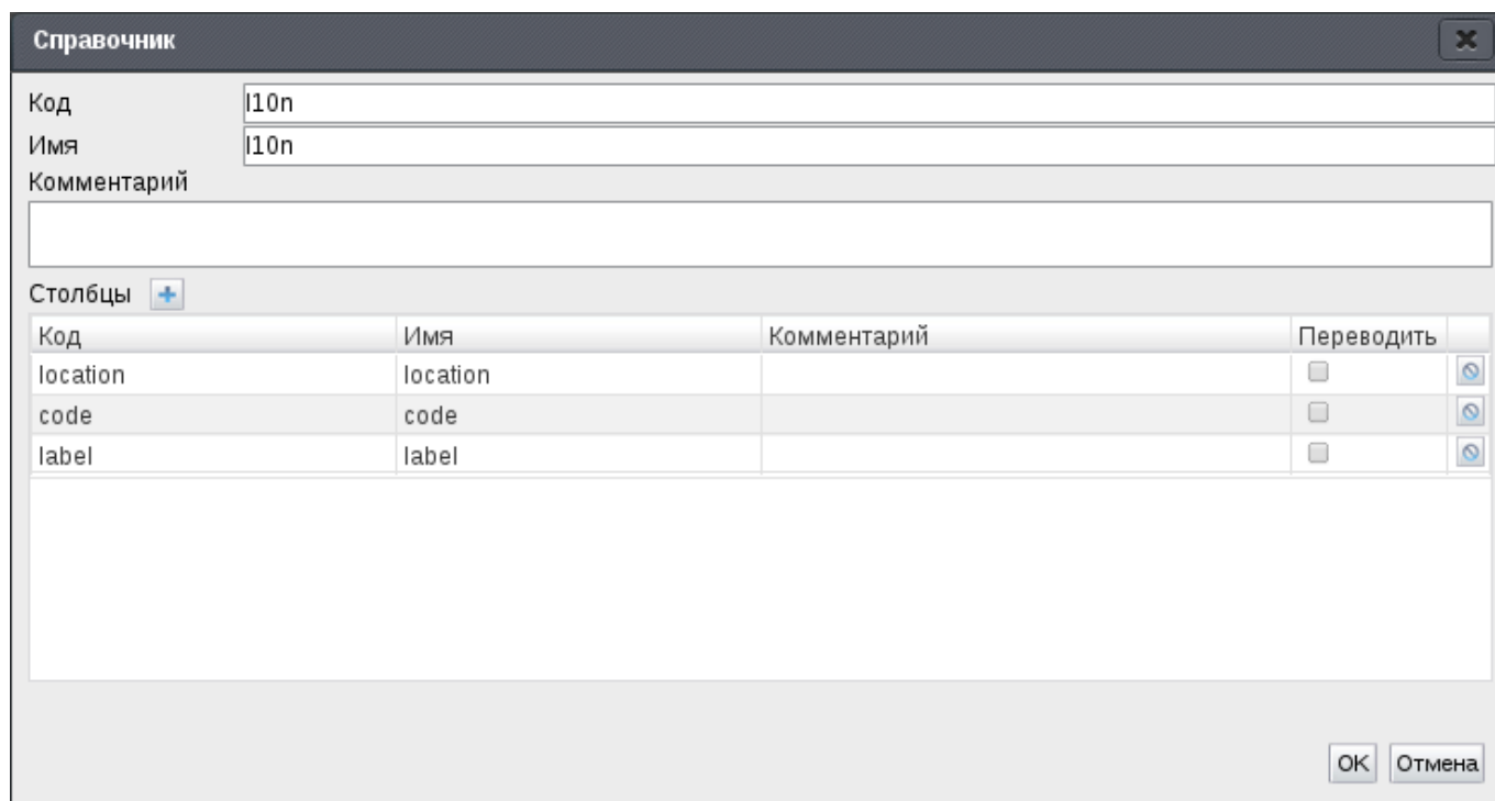
Рис. 3.139: Создание справочника
