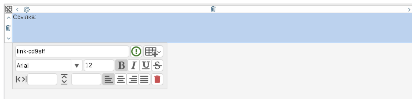
Рис. 3.68: Компонент «Ссылка»
