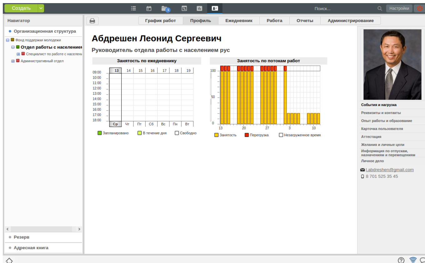
Рис. 5.10: Профиль пользователя
