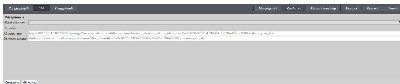
Рис. 3.131: Свойства документа
