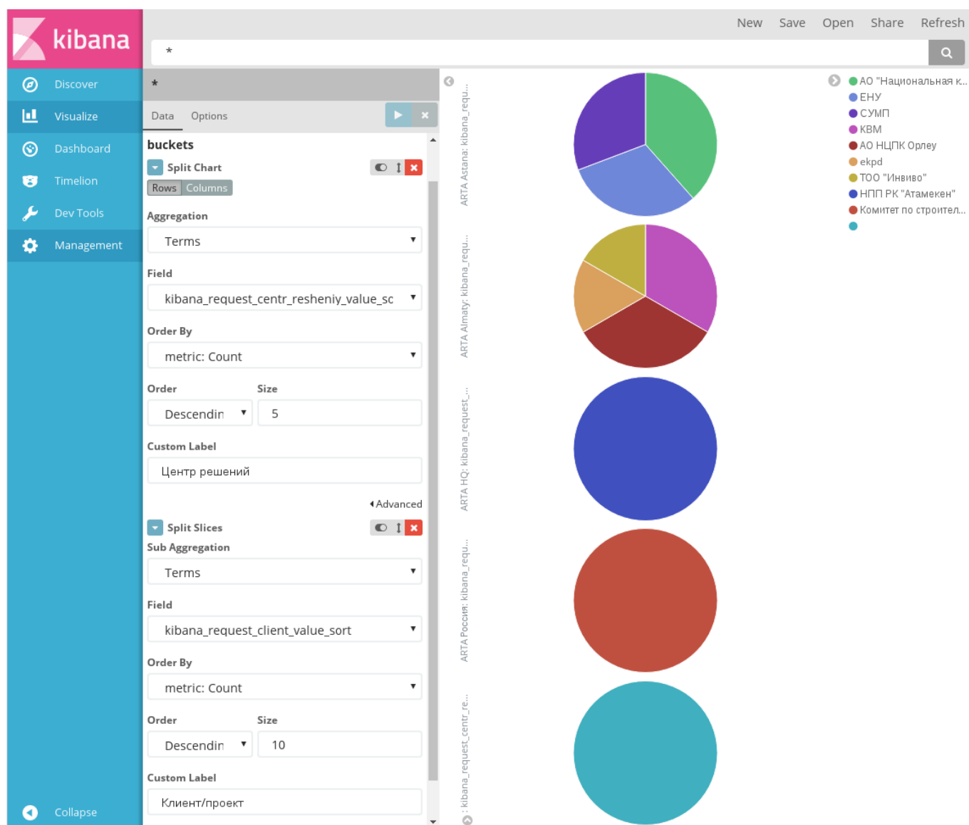
Рис. 1.27: Заявки по офисам и клиентам
