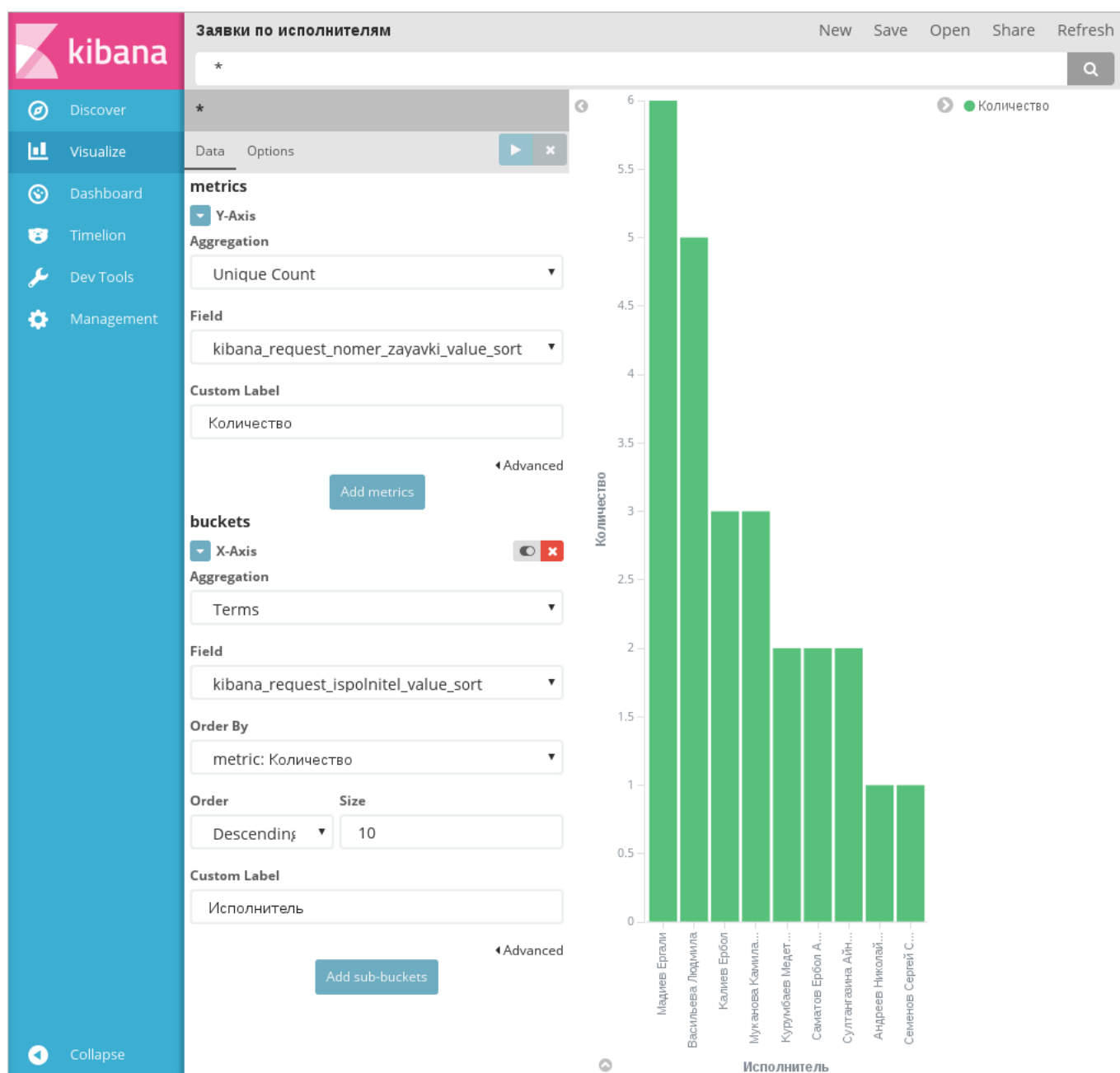
Рис. 1.34: Диаграмма Vertical bar chart, пример 2
