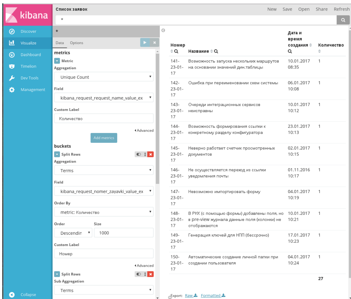
Рис. 1.30: Настроены отображаемые данные в таблице
