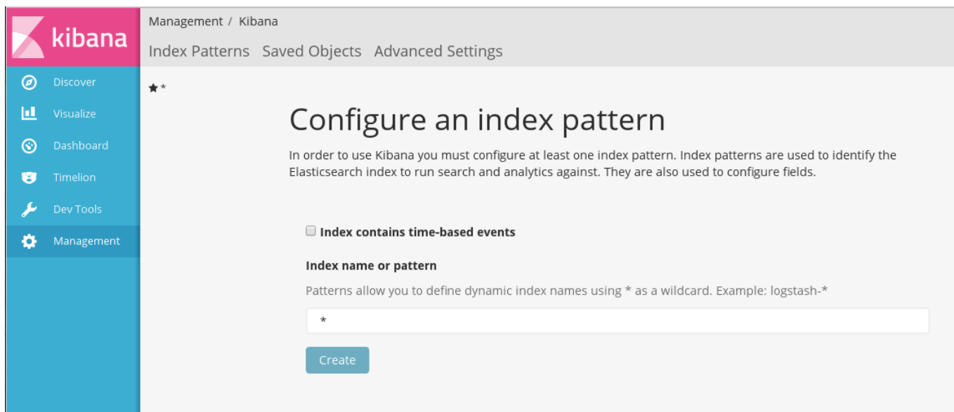
Рис. 1.18: Создание нового шаблона индексов без временных данных
