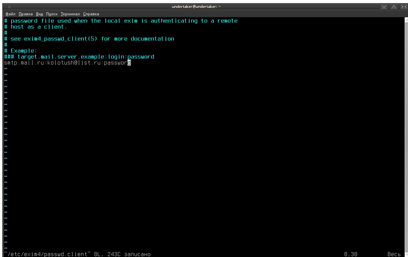
Рис. 7.45: Пример конфигурации аутентификации
