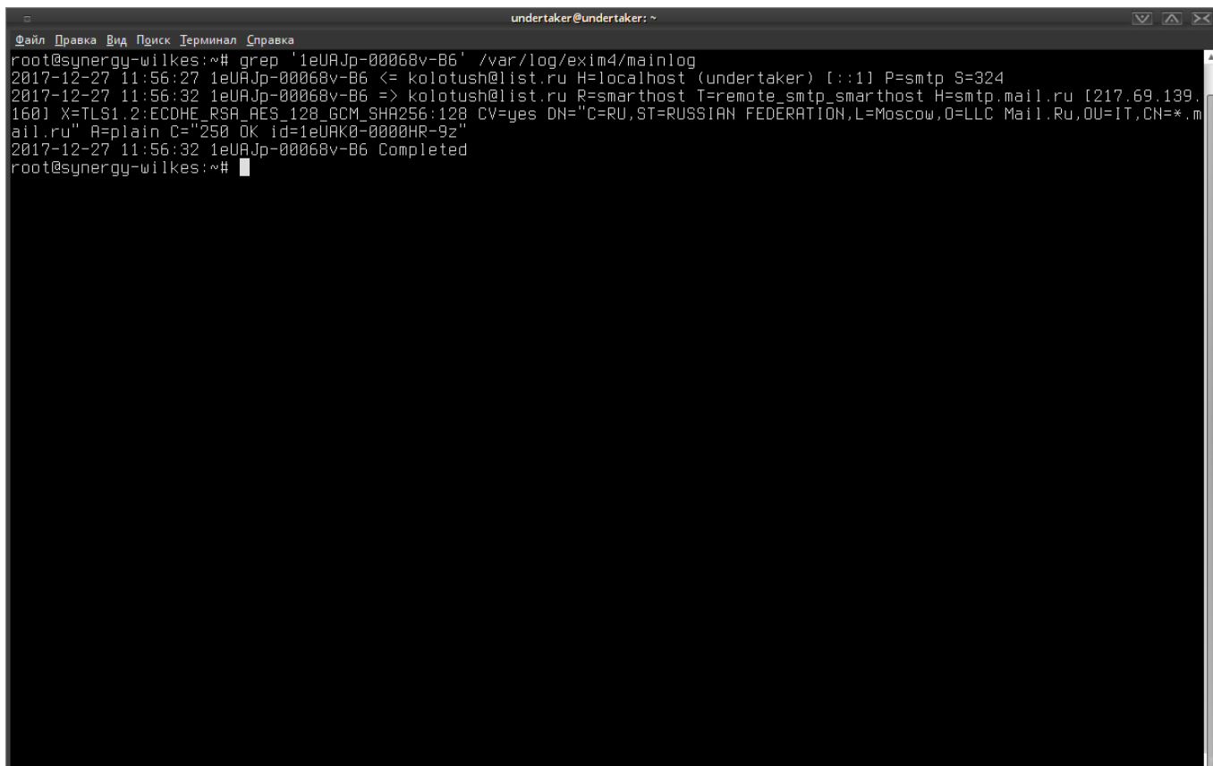
Рис. 7.47: Письмо в логе почтового сервера
