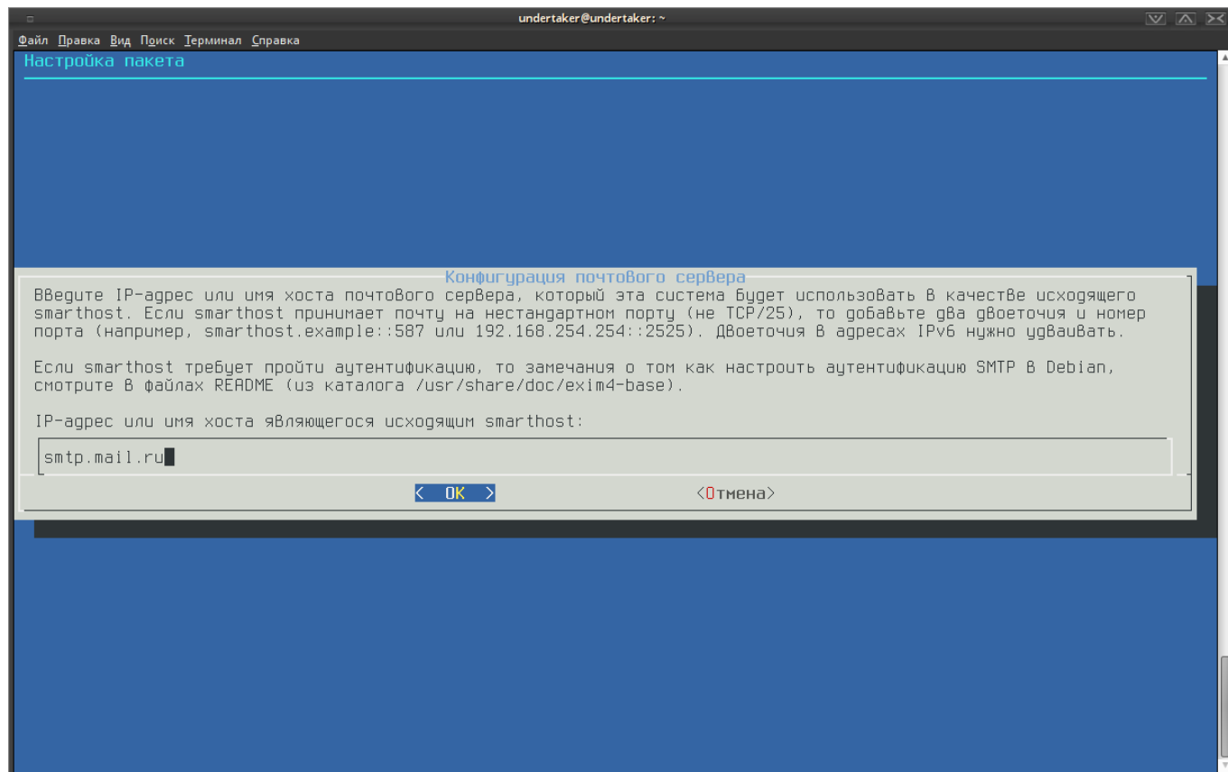
Рис. 7.38: Исходящий почтовый сервер
