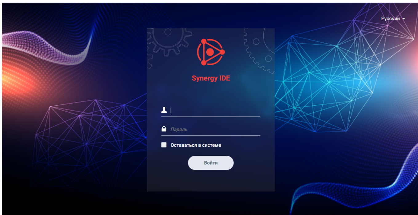
Рис. 2.1: Авторизация
