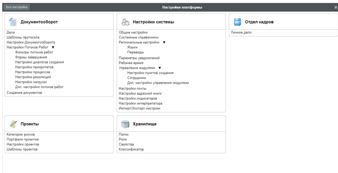
Рис. 2.2: Настройки платформы
