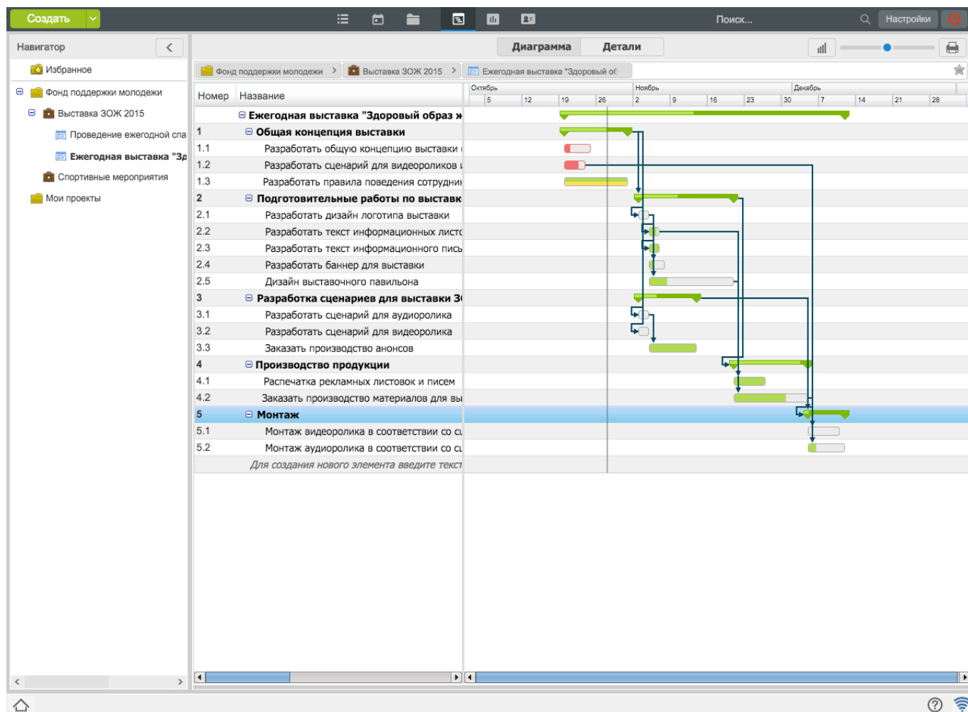
Рис. 8.16: Диаграмма Ганта
